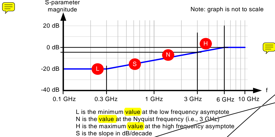
Figure 124 — S-parameter values
