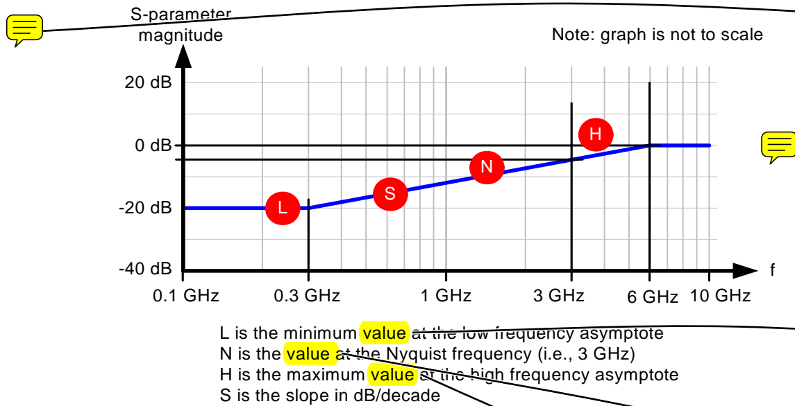
Figure 124 — S-parameter values
